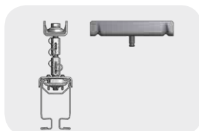
Normal upphängning
